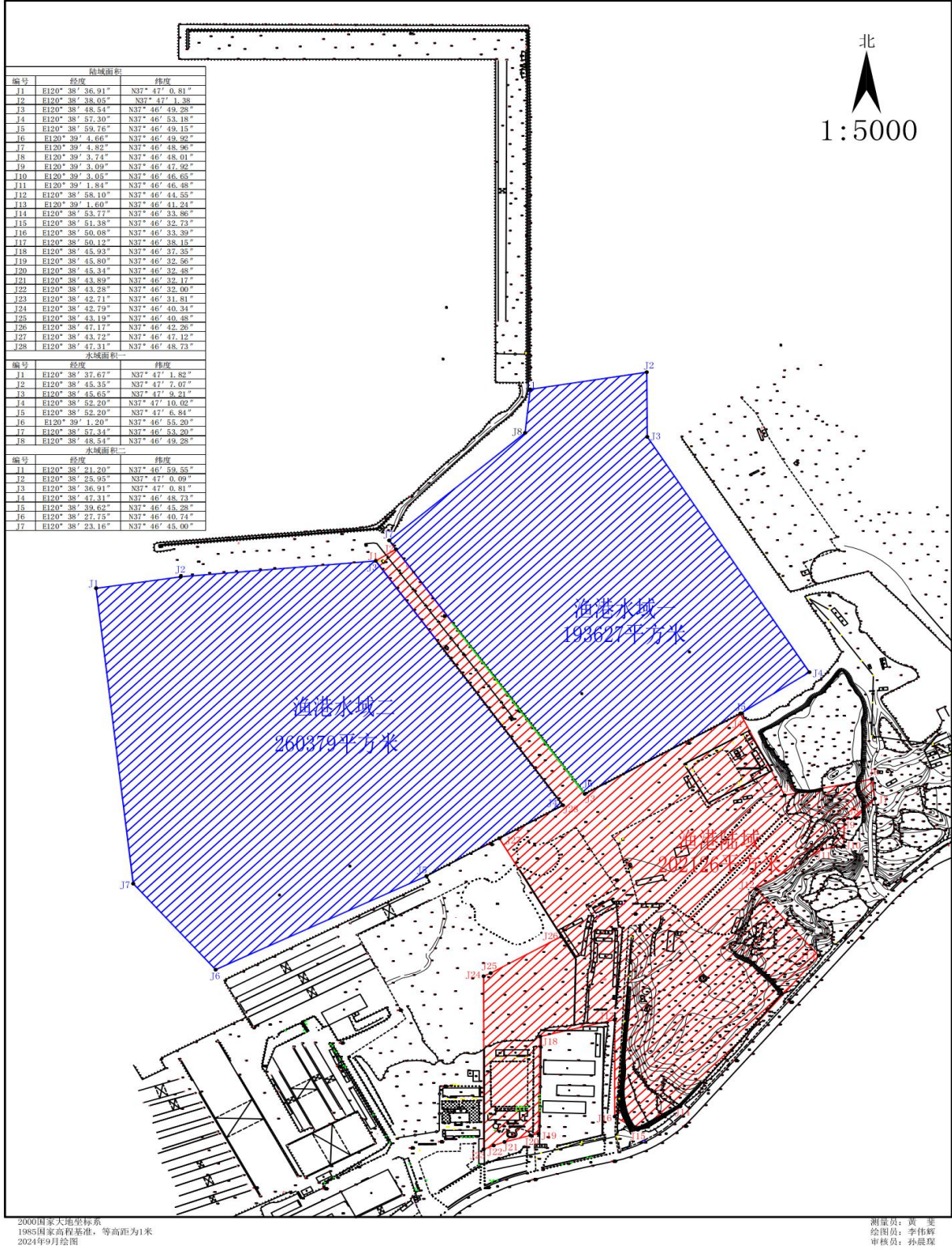
蓬莱渔港港区平面图
